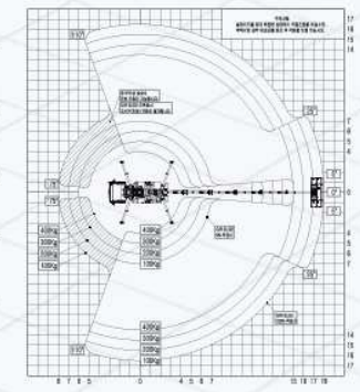
280S 회전방향 작업반경도
